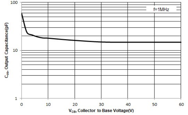
Fig. 6 Output Capacitance
