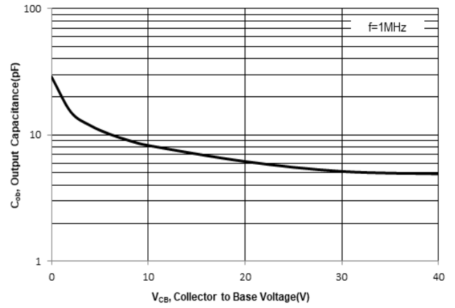
Fig. 6 Output Capacitance
