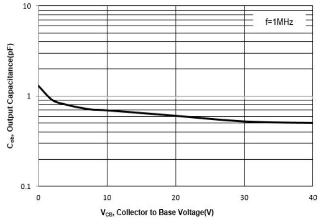
Fig. 6 Output Capacitance
